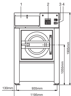
ВИД СПЕРЕДИ FS 33 40 50
