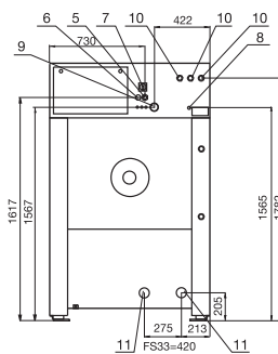
ВИД СЗАДИ FS 33 40 50
